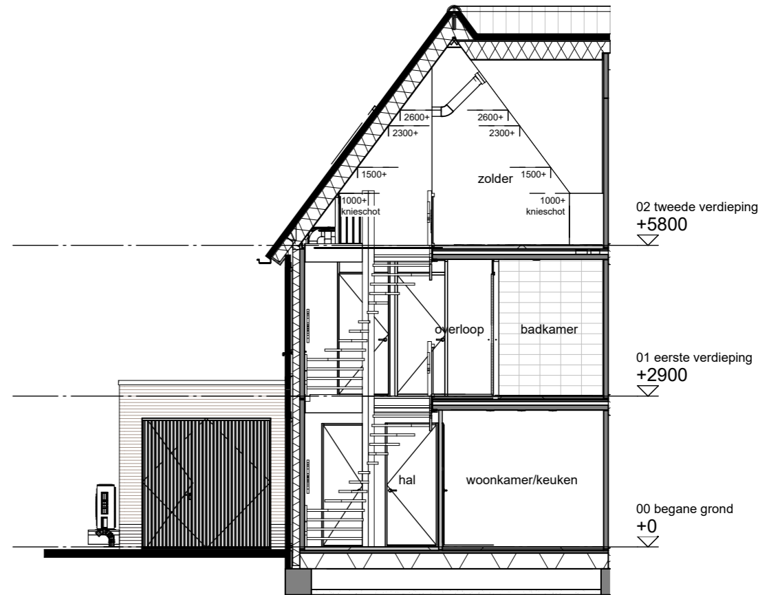
Doorsnede C-C
