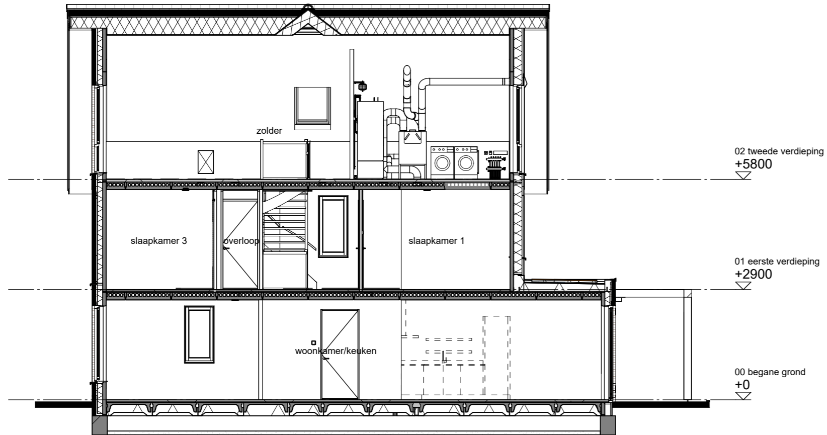
Doorsnede A-A
