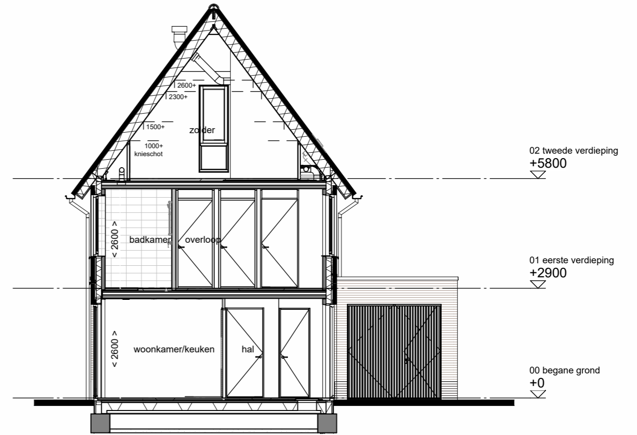
Doorsnede
