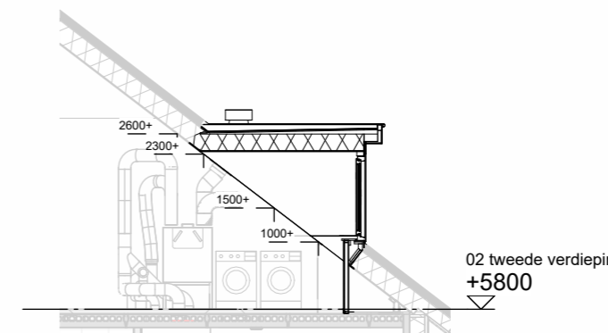
Doorsnede schaal 1:100
