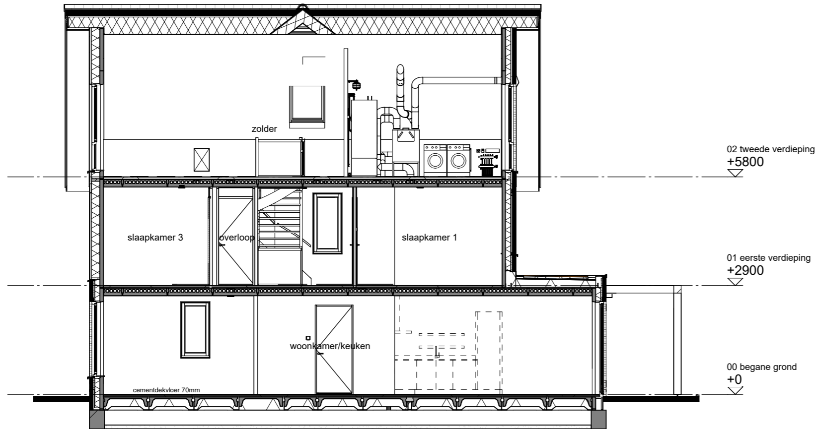
Doorsnede A-A
