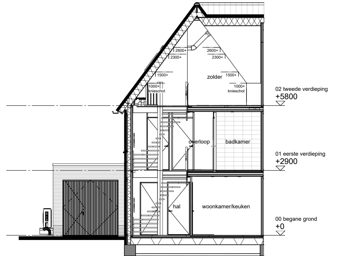
Doorsnede C-C
