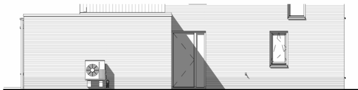
Linkerzijgevel schaal 1:100
