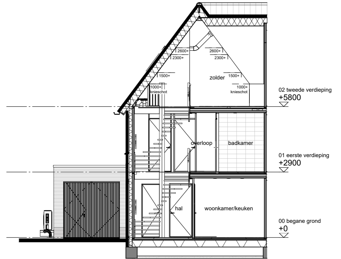
Doorsnede C-C
