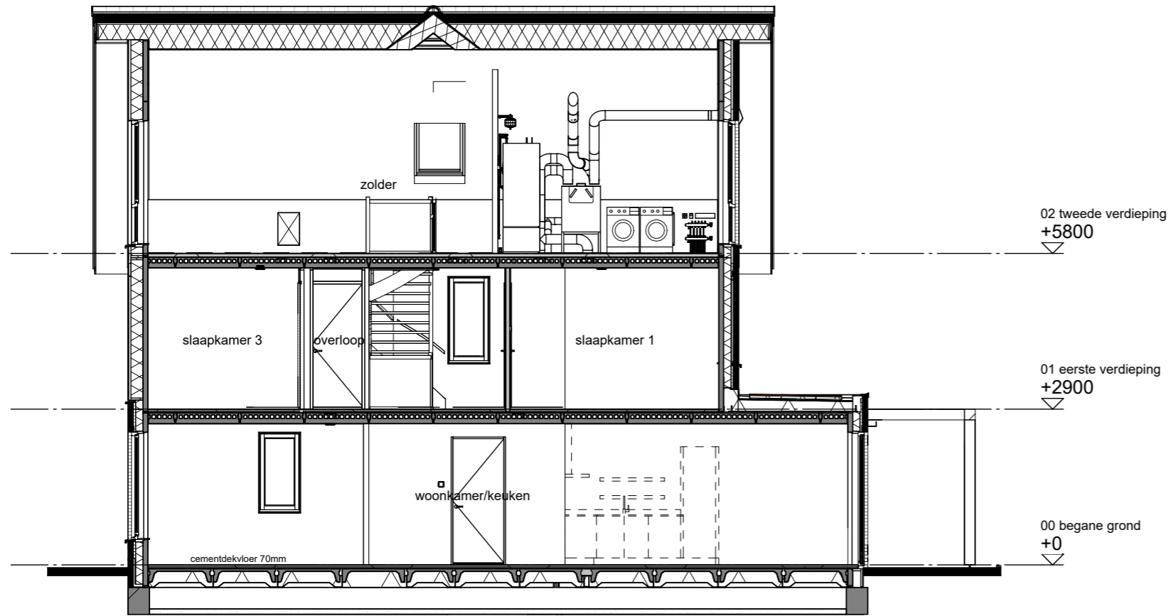
Doorsnede A-A
