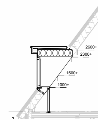
Doorsnede schaal 1:100
