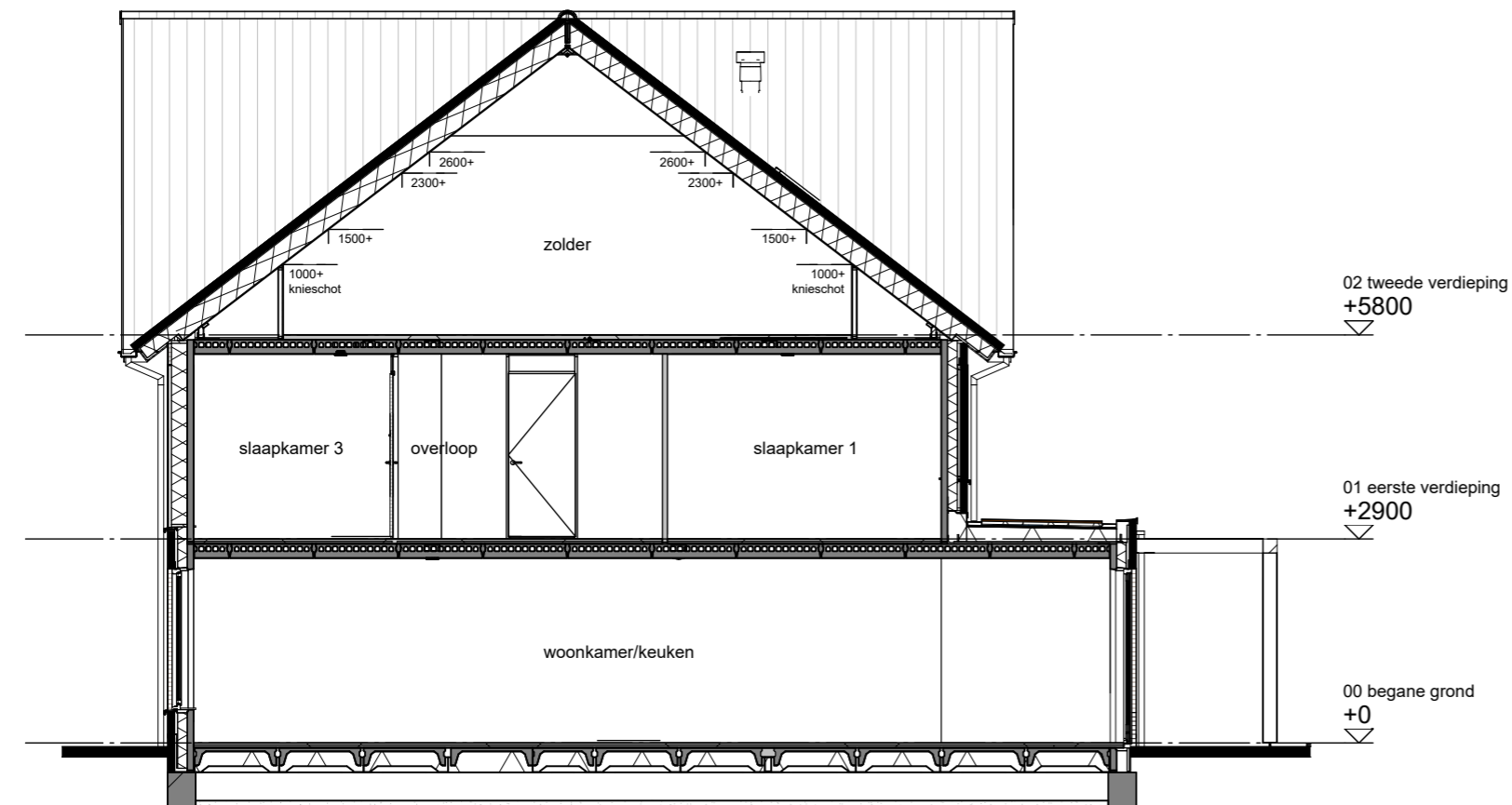
Doorsnede B-B
