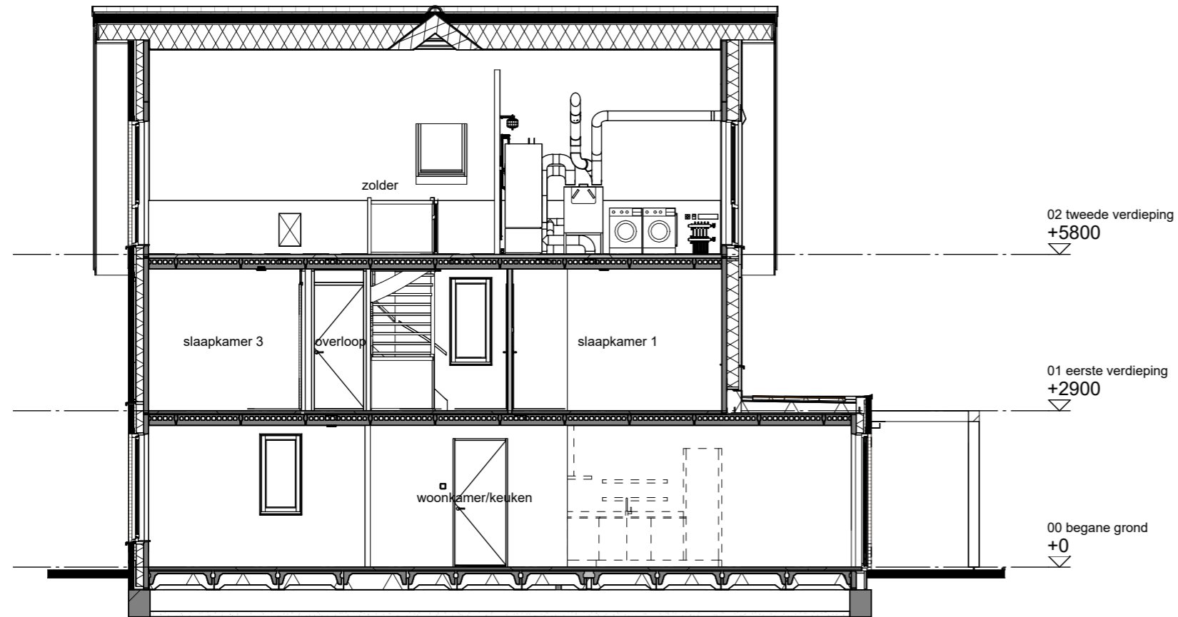
Doorsnede A-A
