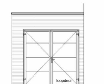
Voorgevel schaal 1:100
