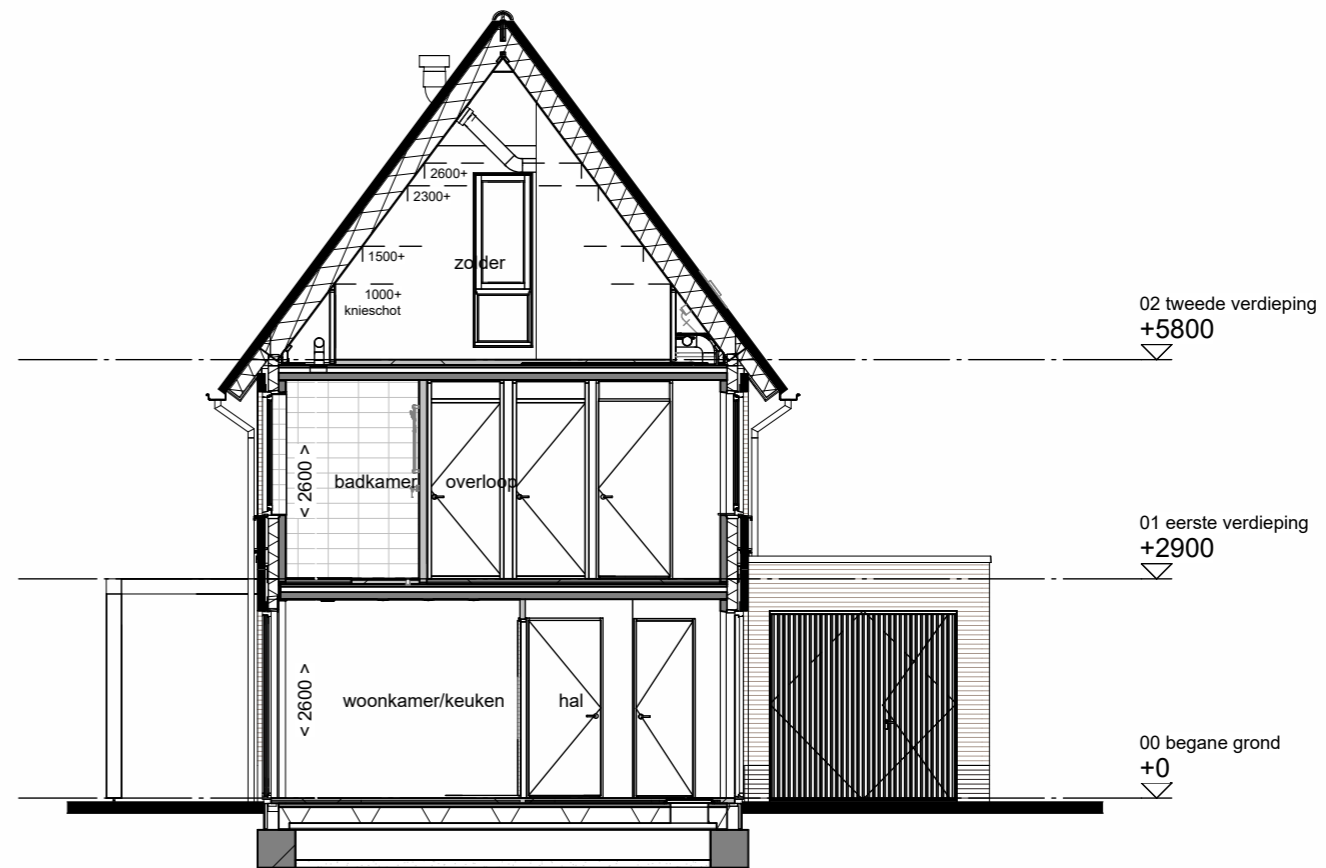
Doorsnede
