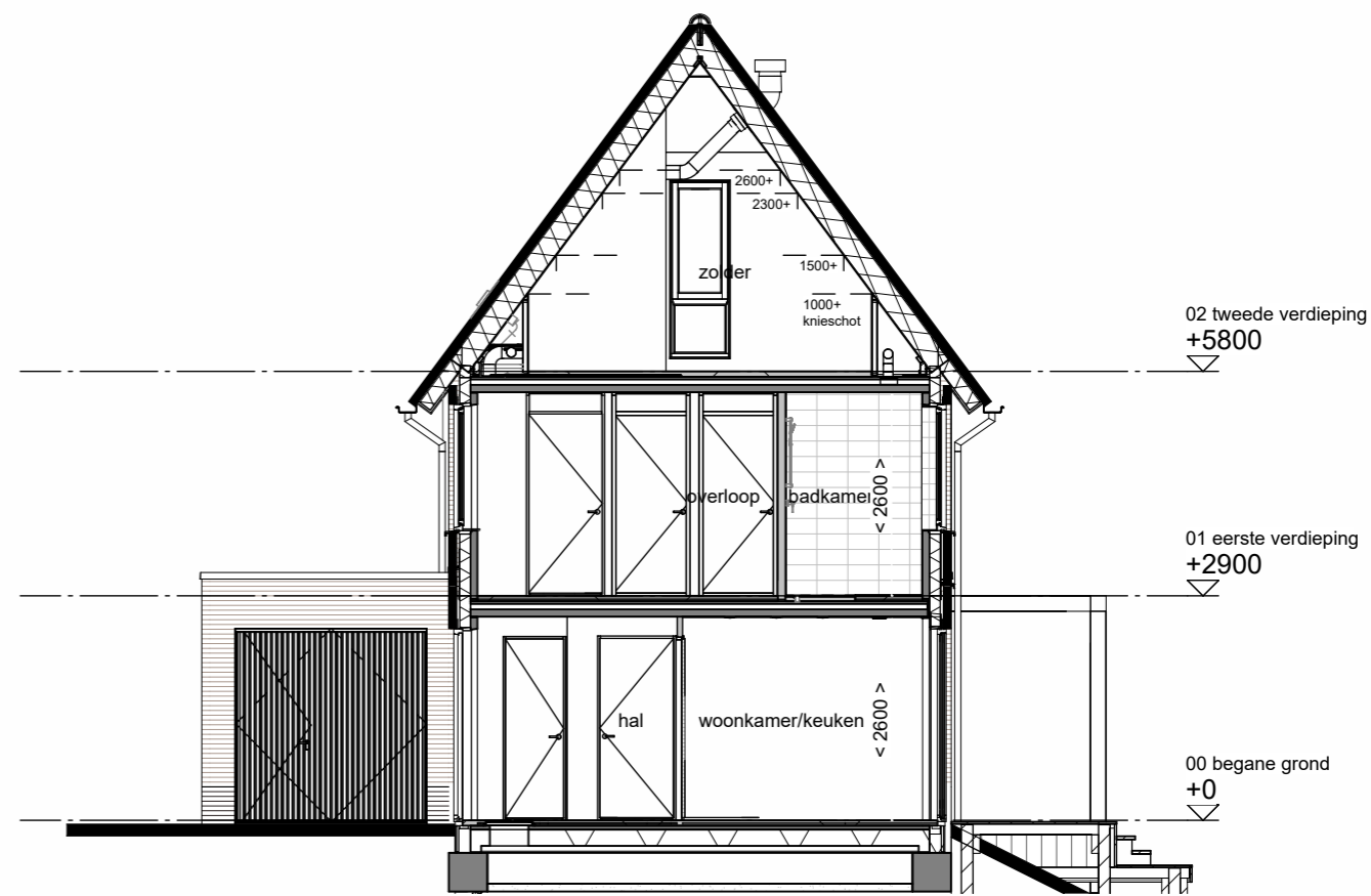
Doorsnede
