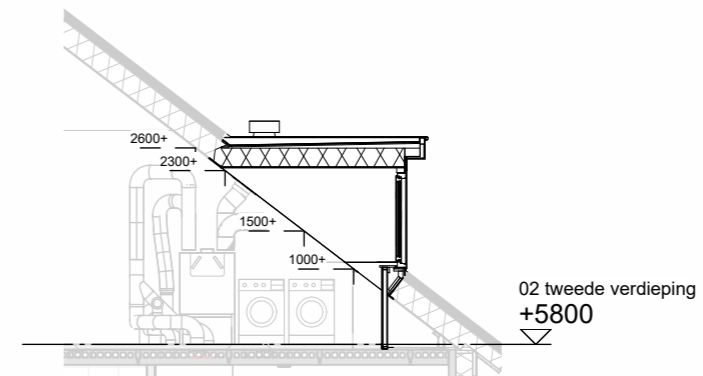
Doorsnede schaal 1:100
