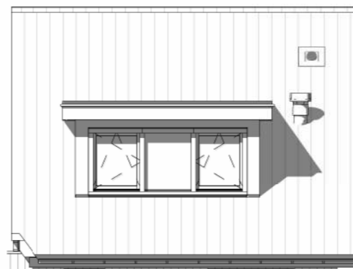
Achtergevel schaal 1:100
