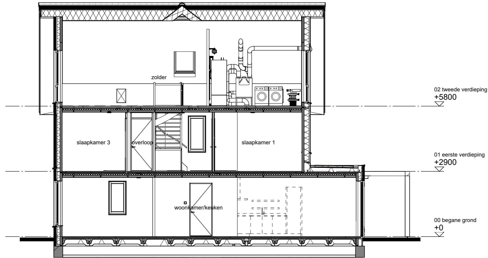
Doorsnede A-A
