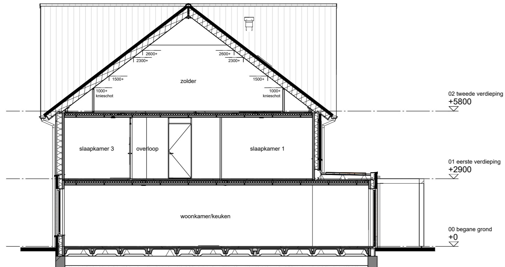
Doorsnede B-B
