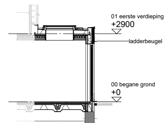
Doorsnede schaal 1:100
