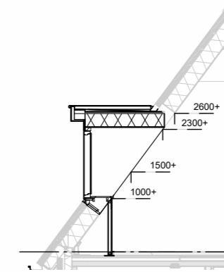
Doorsnede schaal 1:100
