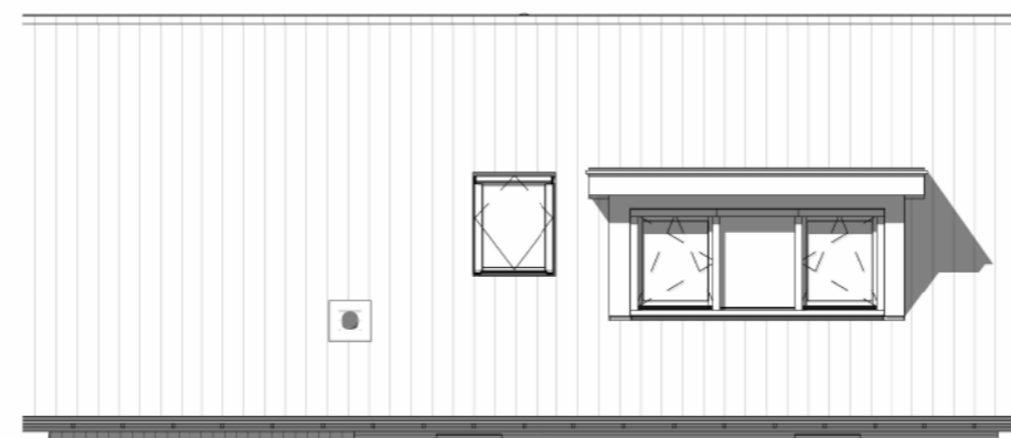
Linkerzijgevel schaal 1:100
