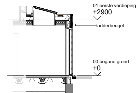
Doorsnede schaal 1:100
