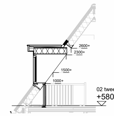
Doorsnede schaal 1:100
