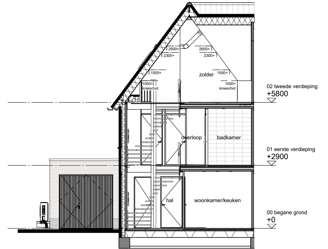
Doorsnede C-C
