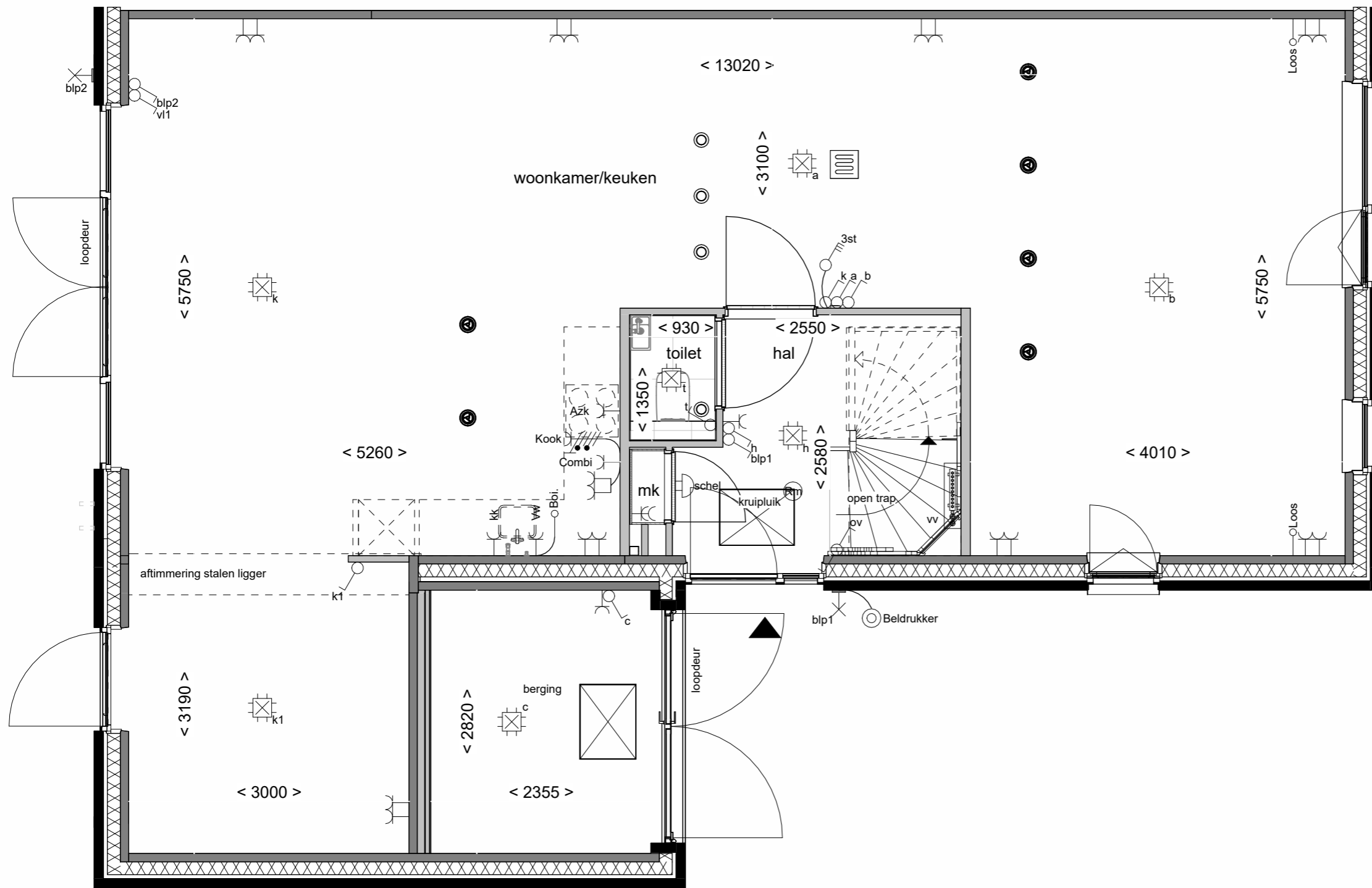
Begane grond
