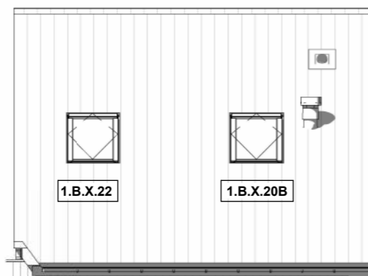
Achtergevel schaal 1:100
