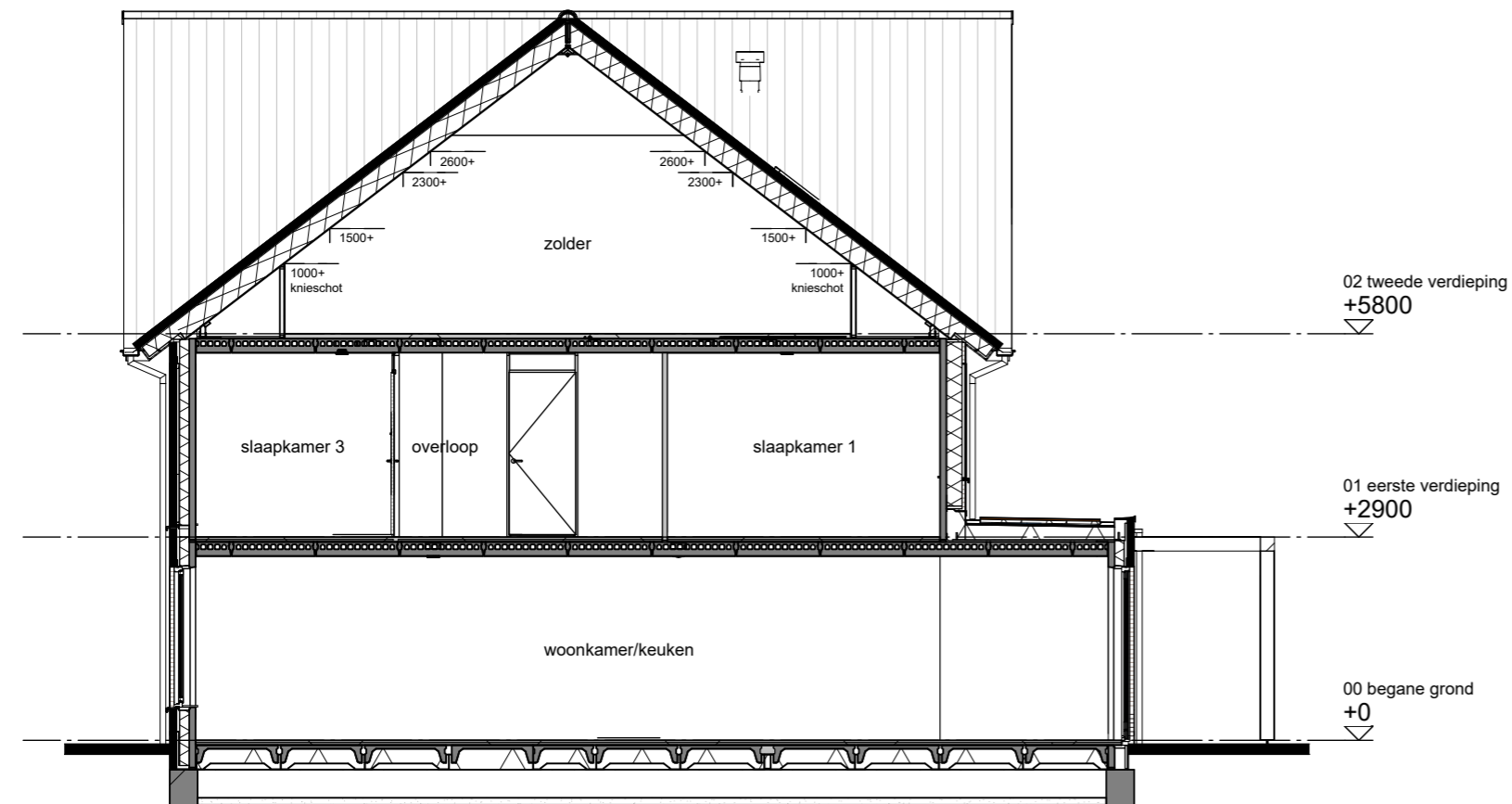
Doorsnede B-B
