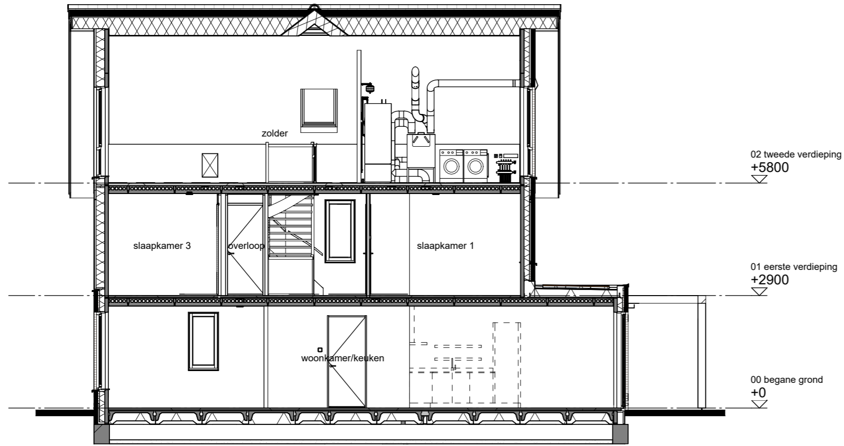
Doorsnede A-A
