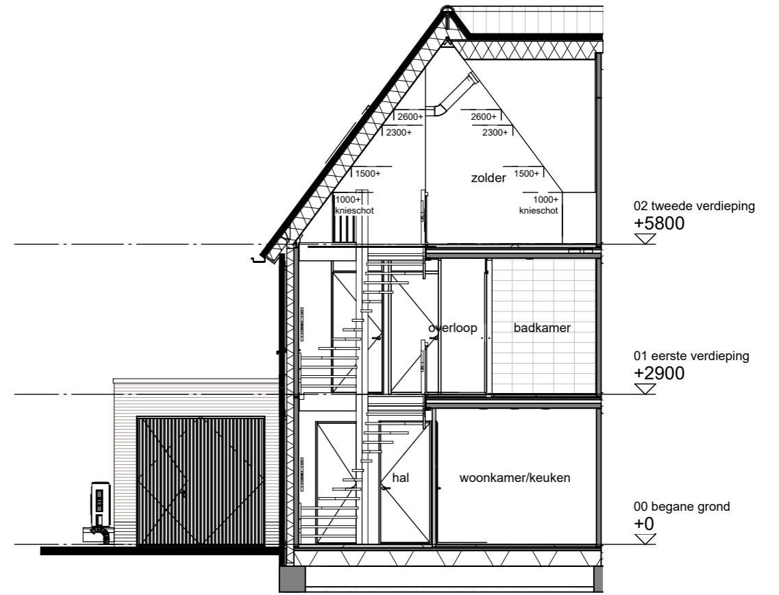
Doorsnede C-C
