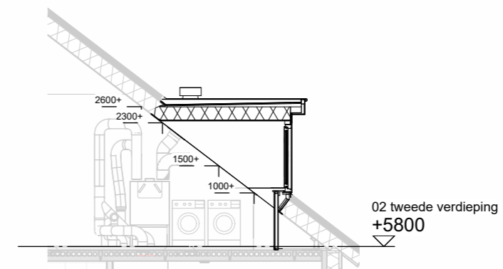
Doorsnede schaal 1:100
