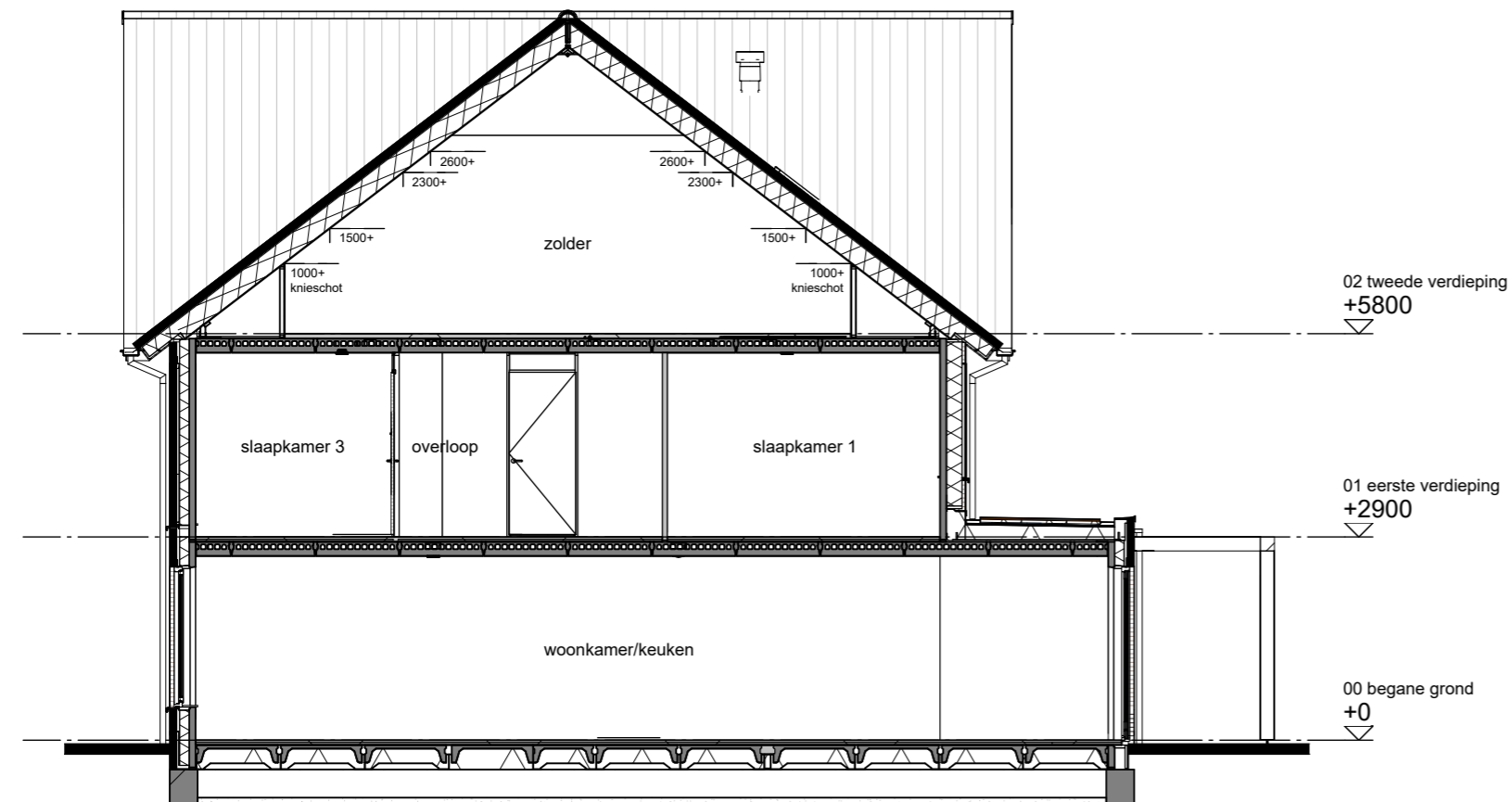
Doorsnede B-B
