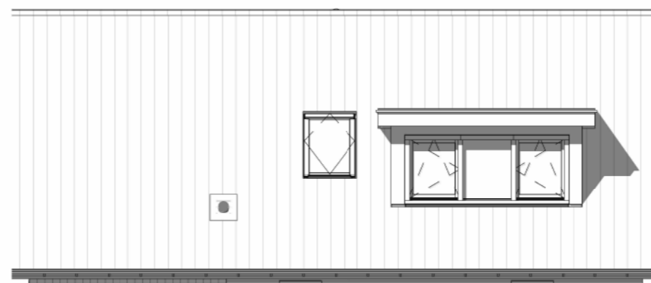
Linkerzijgevel schaal 1:100
