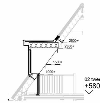
Doorsnede schaal 1:100
