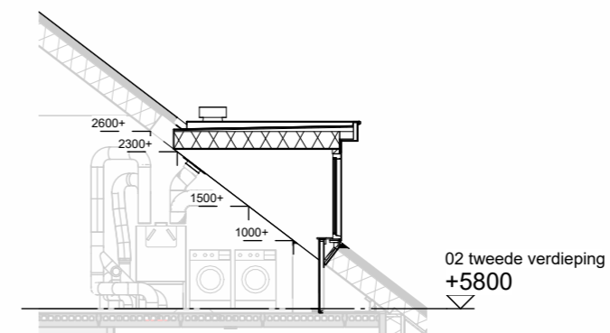
Doorsnede schaal 1:100
