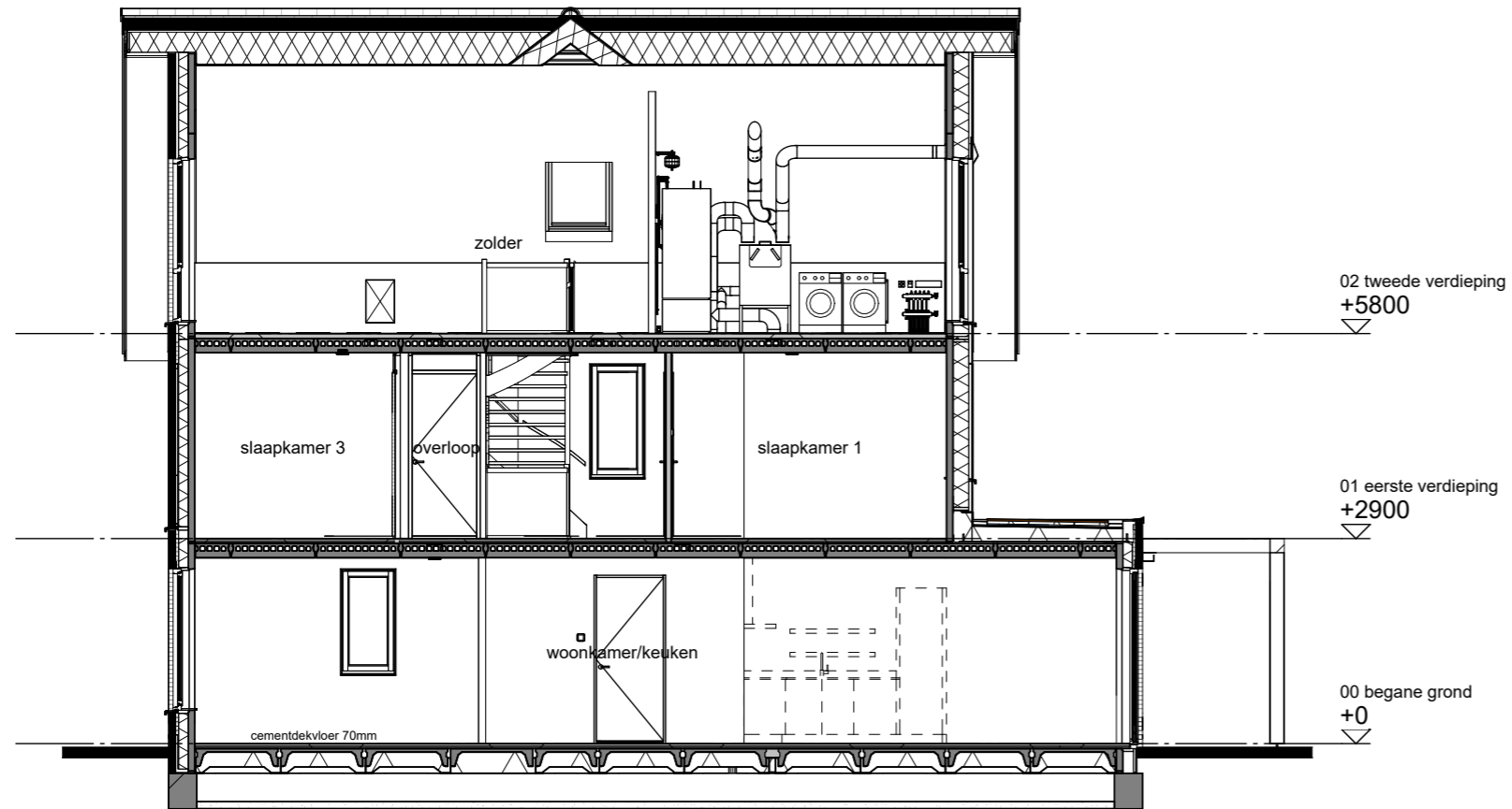
Doorsnede A-A
