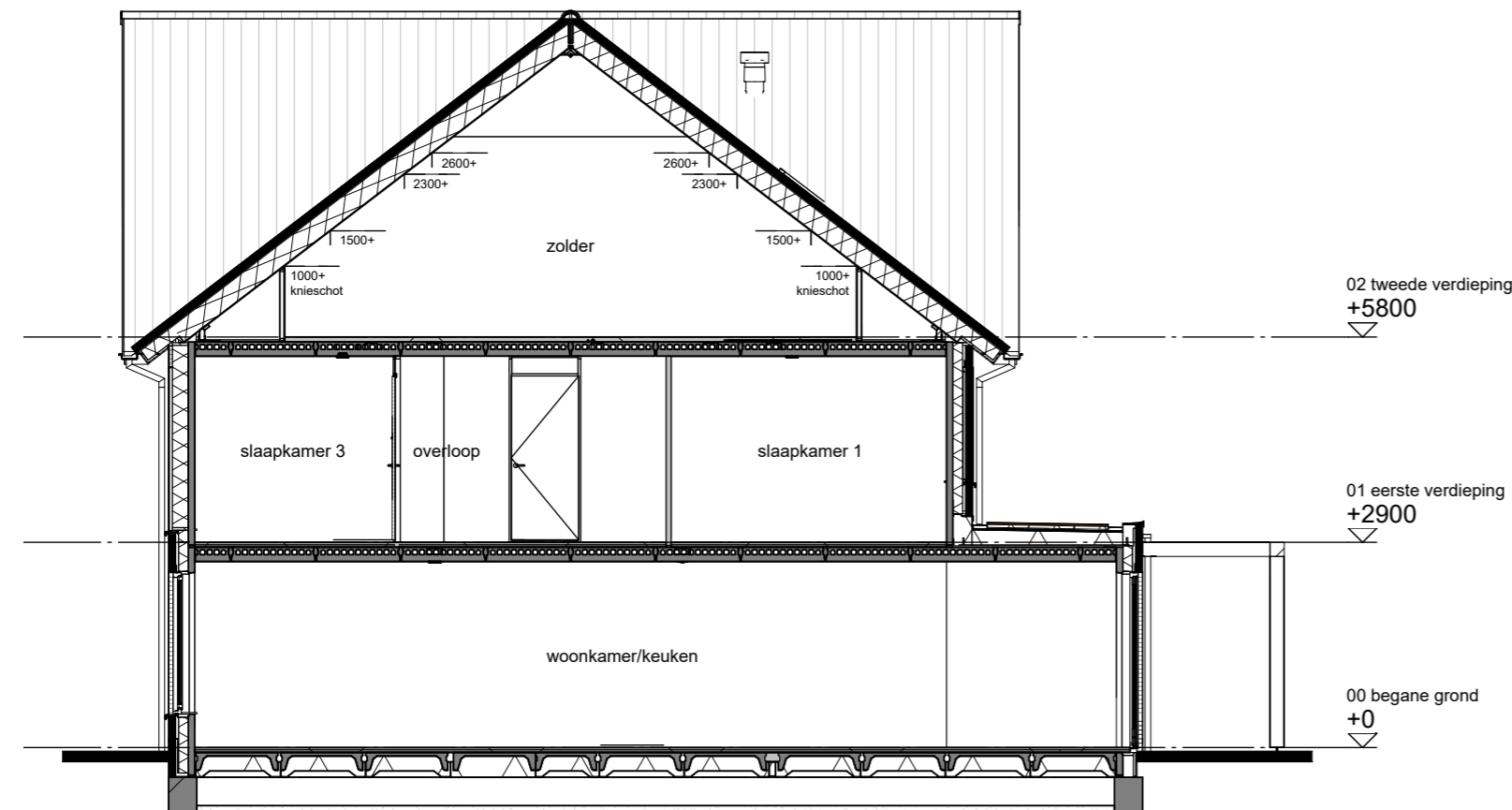
Doorsnede B-B
