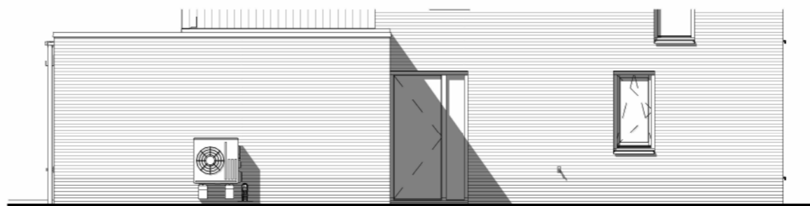
Linkerzijgevel schaal 1:100
