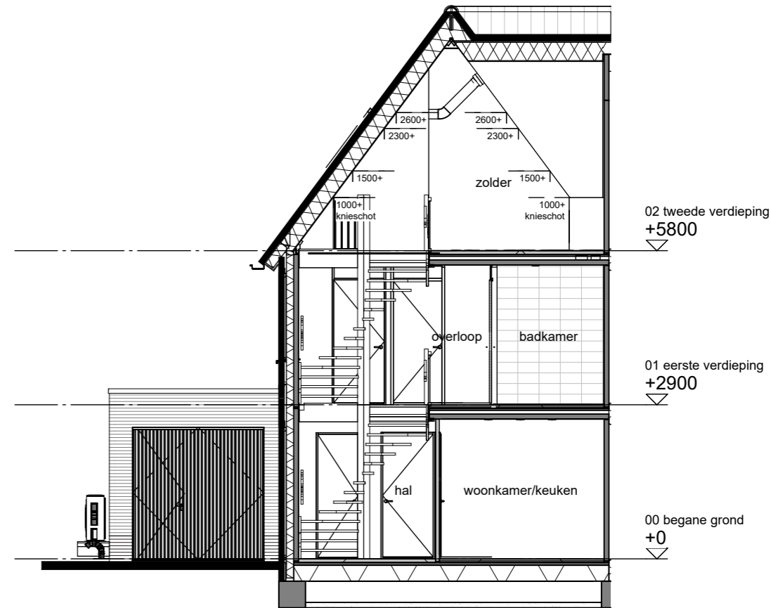
Doorsnede C-C
