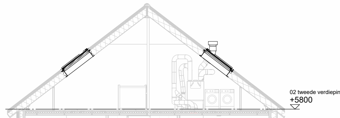
Doorsnede schaal 1:100
