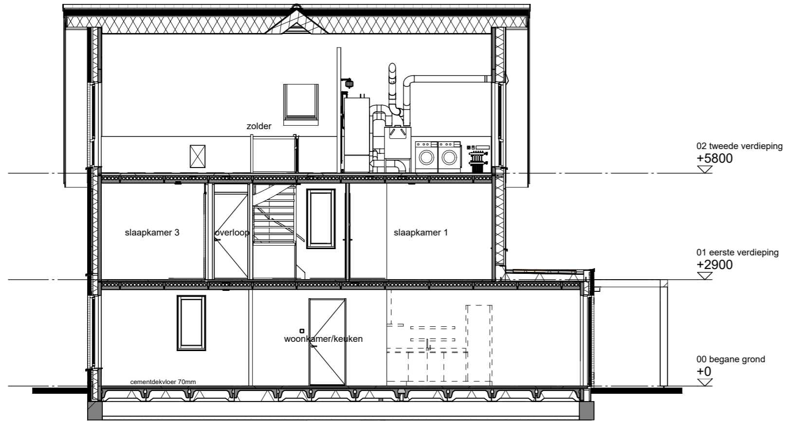
Doorsnede A-A
