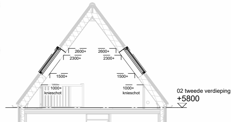
Doorsnede schaal 1:100
