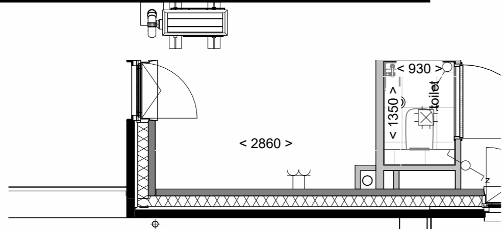
Eerste verdieping (extra schacht)
