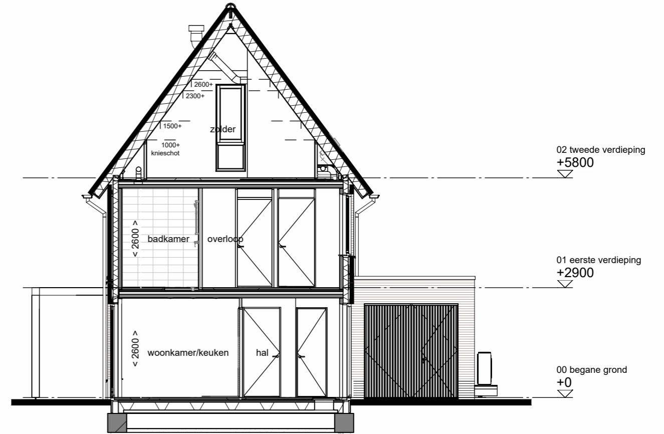
Doorsnede
