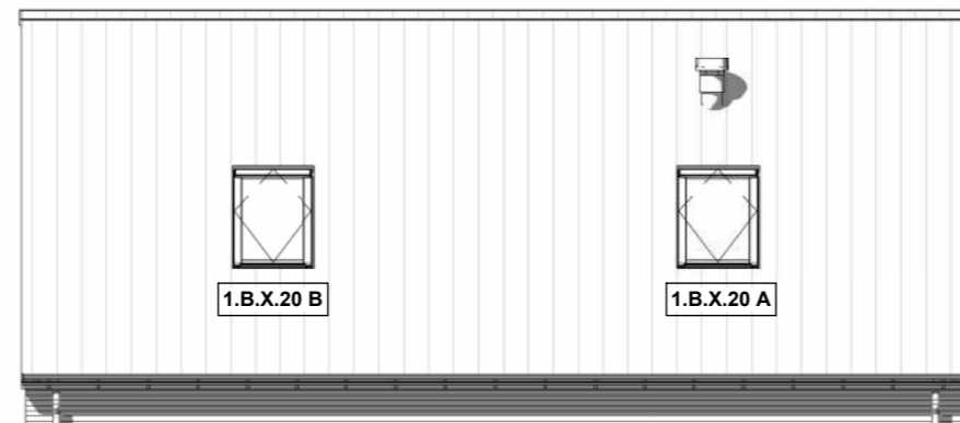
Rechterzijgevel schaal 1:100
