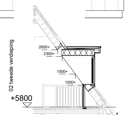
Doorsnede schaal 1:100
