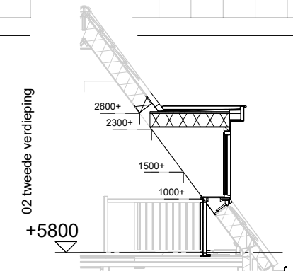
Doorsnede schaal 1:100
